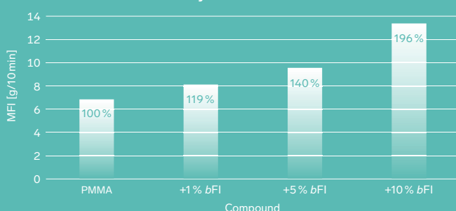
Fließverbessernde Eigenschaften von Polytives bFI in PMMA
